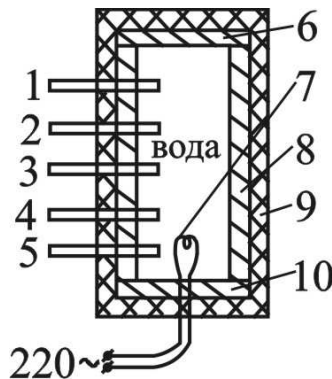
Рисунок 3.1 - Схема установки для исследования конвективного теплообмена в воде: 1, 2, 3, 4, 5 - термометры; 6 - фланец верхний; 7 - нагревательный элемент; 8 - труба; 9 - теплоизоляция; 10 - фланец нижний
