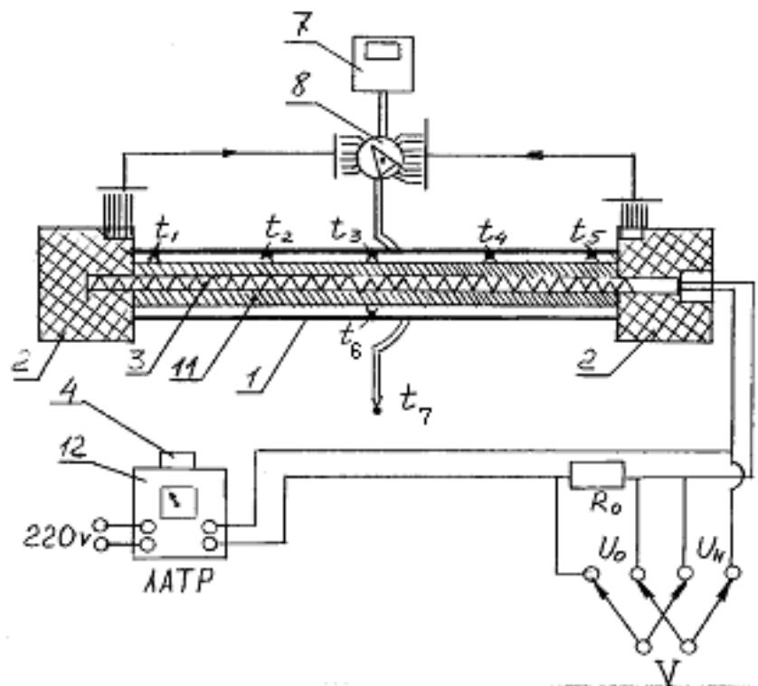
Рисунок 4.1 – Лабораторная установка: 1 – медная тонкостенная труба; 2 - заглушка из теплоизолирующего материала; 3 – нагреватель; 4 – регулятор ЛАТРа; 5 – мультиметр; 6 - переключатель мультиметра; 7 – измеритель температуры; 8 – переключатель измерения температуры; 9 – тумблер; 10 – тумблер включения нагревателя; 11 – термостат; 12 - источник переменного напряжения (ЛАТР)
