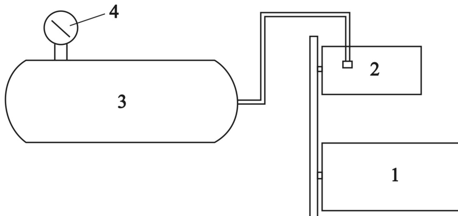
Рисунок 6.1 - Схема установки для исследования компрессора: 1 – электродвигатель; 2 – компрессор; 3 – ресивер; 4 - манометр
